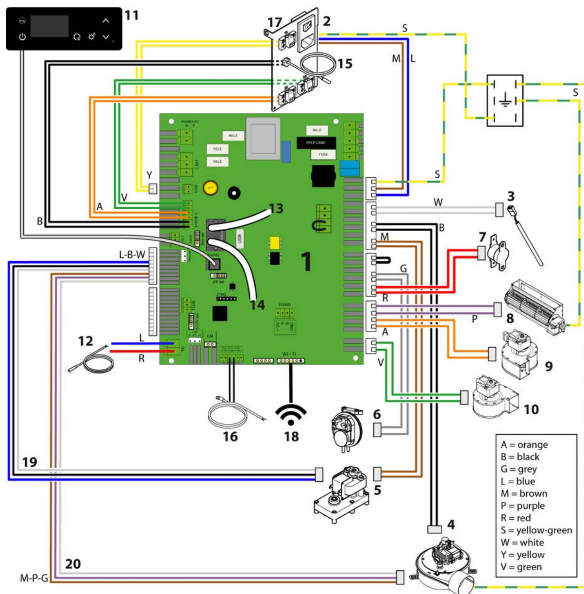
OBJAŚNIENIE SCHEMATU MONTAŻOWEGO ZESPOŁU
